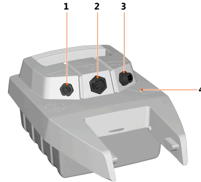
Fig. 81: Overzicht accu
