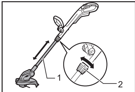
► 1. Shaft 2. Grip
