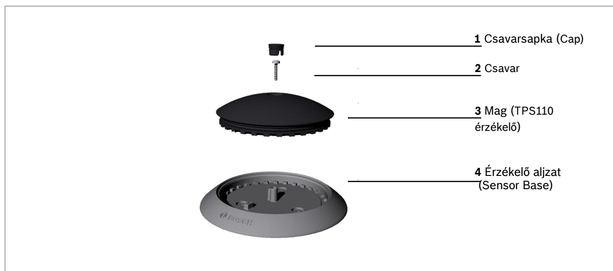
1. ábra: TPS110 érzékelőmaggal ellátott PLS parkolóérzékelő
