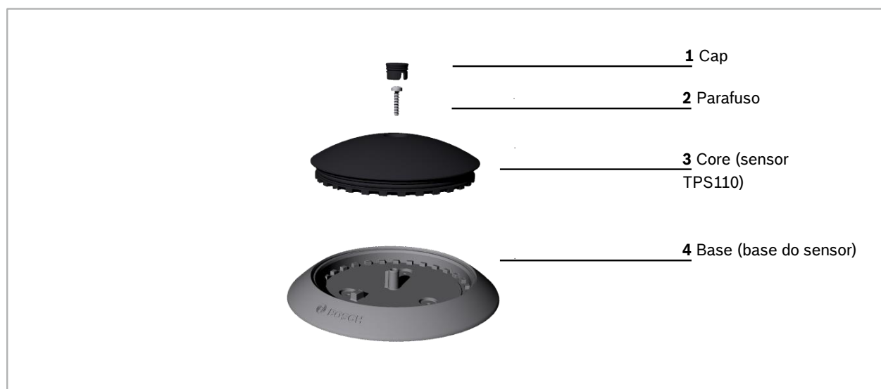
Figura 1 Sensor de estacionamento PLS com núcleo de sensor TPS110
