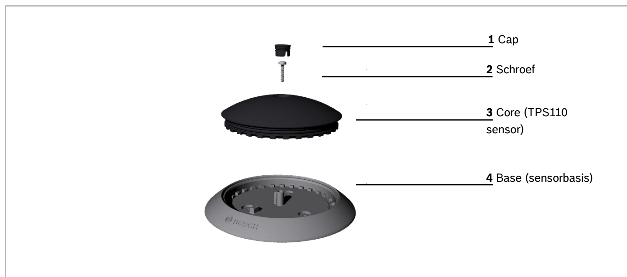
Afbeelding 1 Parking Lot Sensor PLS met TPS110 sensorkern
