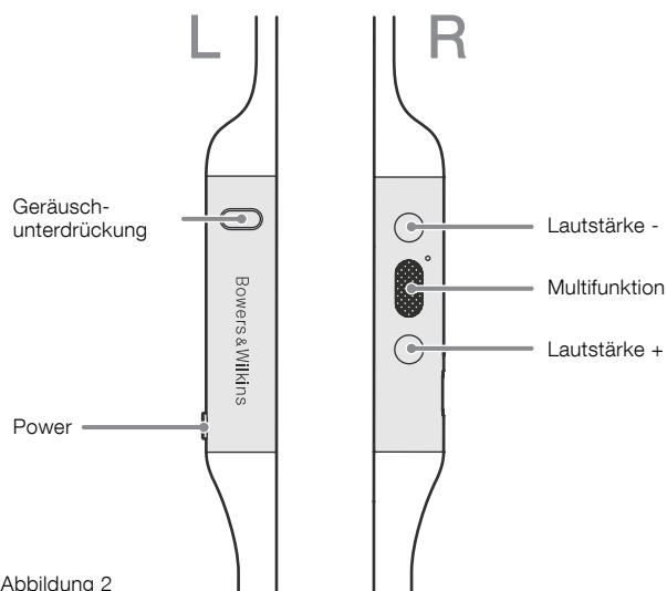
Abbildung 2 Kopfhörer-Bedienelemente
