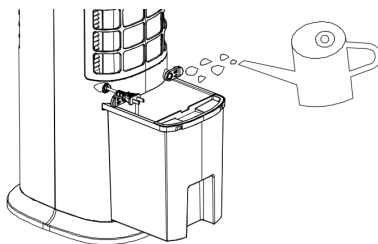
Retirez le réservoir pour le remplir d'eau
