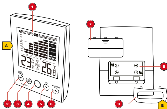
Abb. 1: Teileübersicht für das Hygrometer
