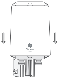
Montage mural
