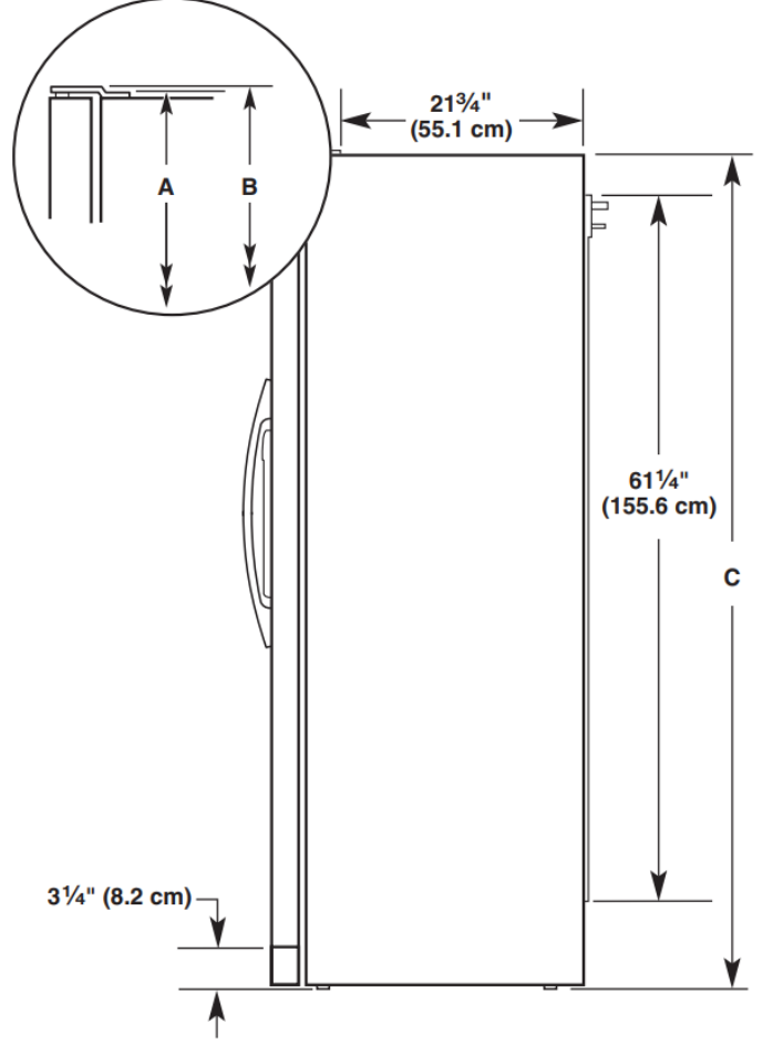
Dimensions du produit – Vue latérale
