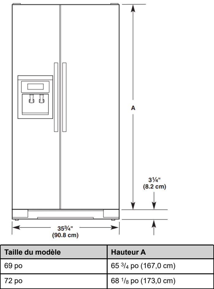
Dimensions du produit – Vue avant
