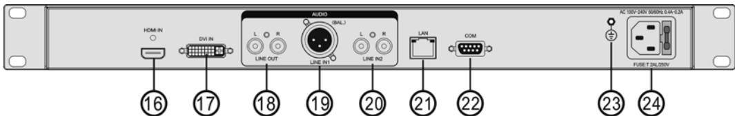
HCS-8316HDMI 后面板
