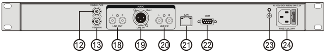
HCS-8316AV-H 后面板
