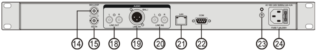
HCS-8316SDI 后面板
