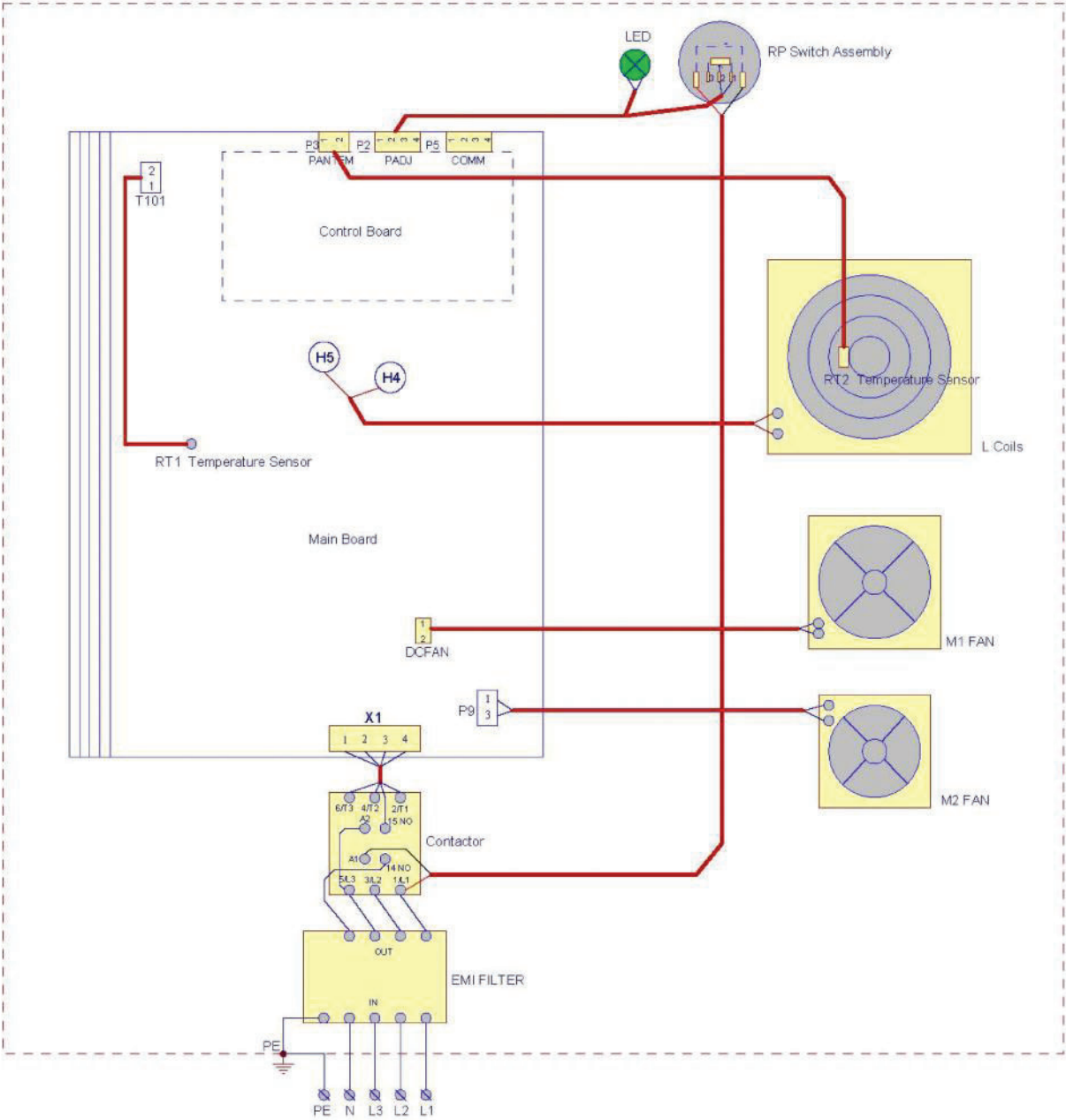
Kytentäkaavio / Kopplingsschema / Wiring diagram 5 kW
