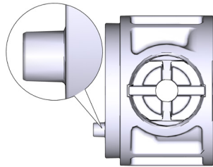
Pressure Balance Puck (F6) Disco de equilibrio de presión (F6) Rondelle d'équilibrage de pression (F6)
