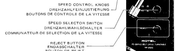
Fig. 8 Control Panel Abb. 8 Bedienungsfeld Fig. 8 Paneau de Contrôle
