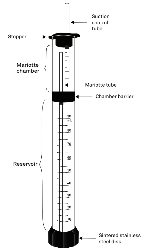
Figure 5 Mini Disk Infiltrrometer diagram
