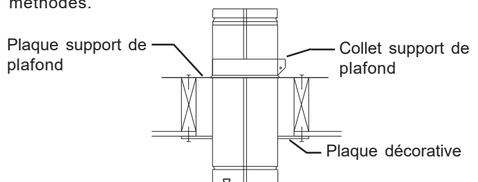
Schéma 3 Support de plafond
