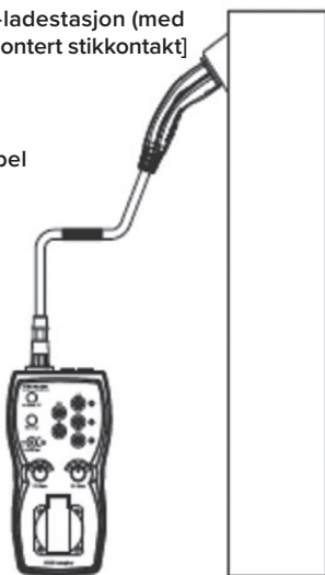
Tilkobling av testadapteren til en type 2-ladestasjon med panelmontert stikkontakt
