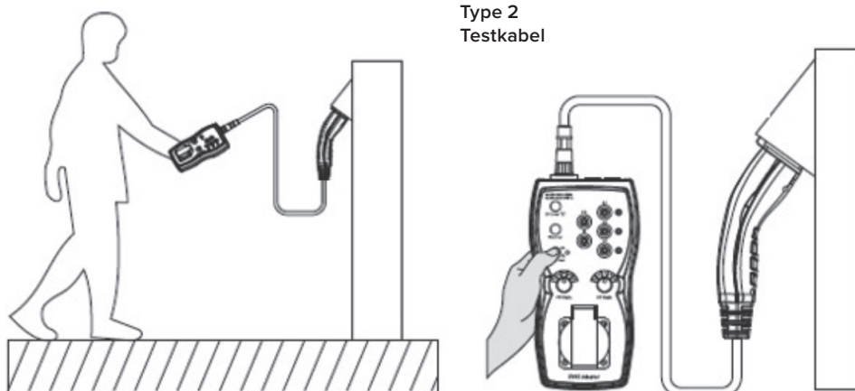
Type 2-ladestasjon (med panelmontert stikkontakt)
