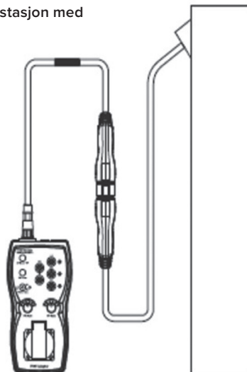
Tilkobling av testadapteren til en type 2-ladestasjon med fast kabel og kjøretøykontakt
