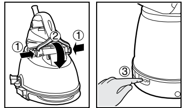
Fig. 4: Ontgrendelen en aanzetten van het striksysteem.
