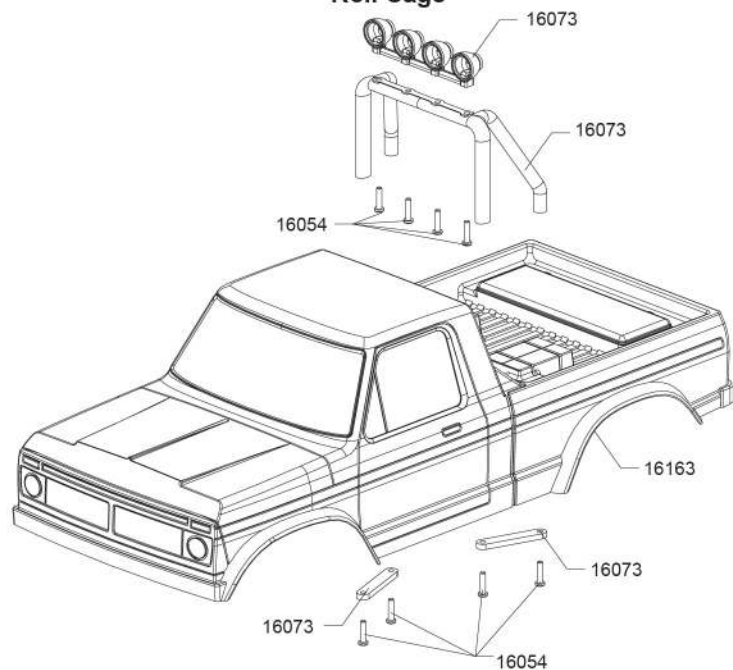
Roll Cage
