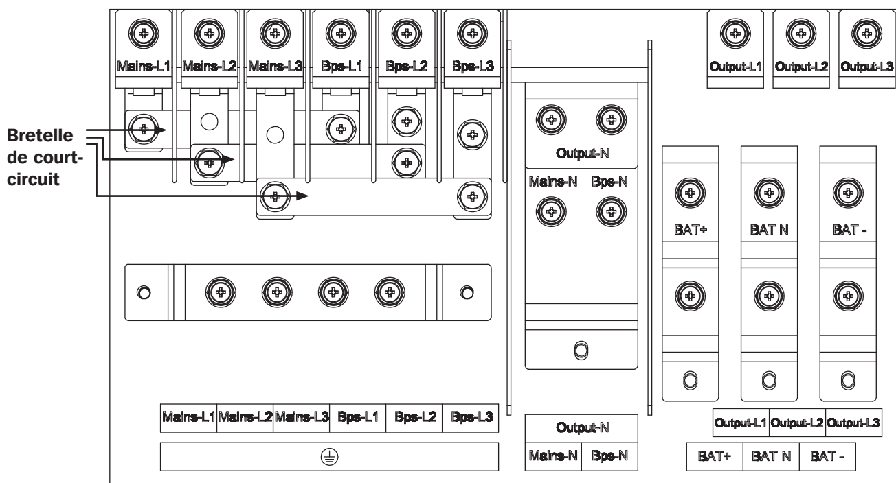
Figure 3-11 : connexion d'entrée simple, modèles S3M50K et S3M60K
