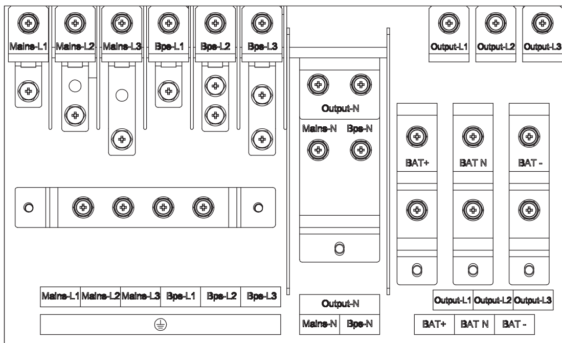
Figure 3-14 : connexion d'entrée double, modèles S3M50K et S3M60K
