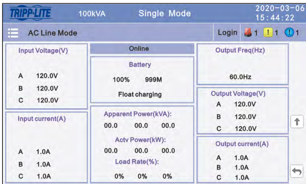
Figura 4-7B: Página Principal del LCD 2. (Presione el Ícono Page Up [página hacia arriba] para regresar a la página principal que se muestra en la Figura 4-7A).
