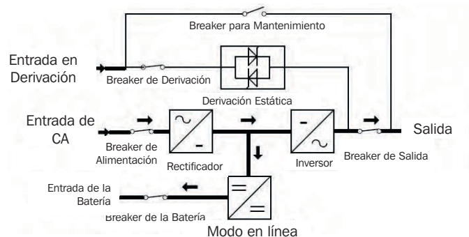
Figura 4-1: Modo en Línea de CA
