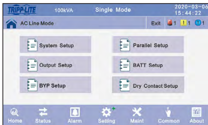
Figura 4-27: Interfaz de Configuraciones Avanzadas
