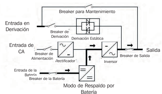
Figura 4-2: Modo de Respaldo por Batería
