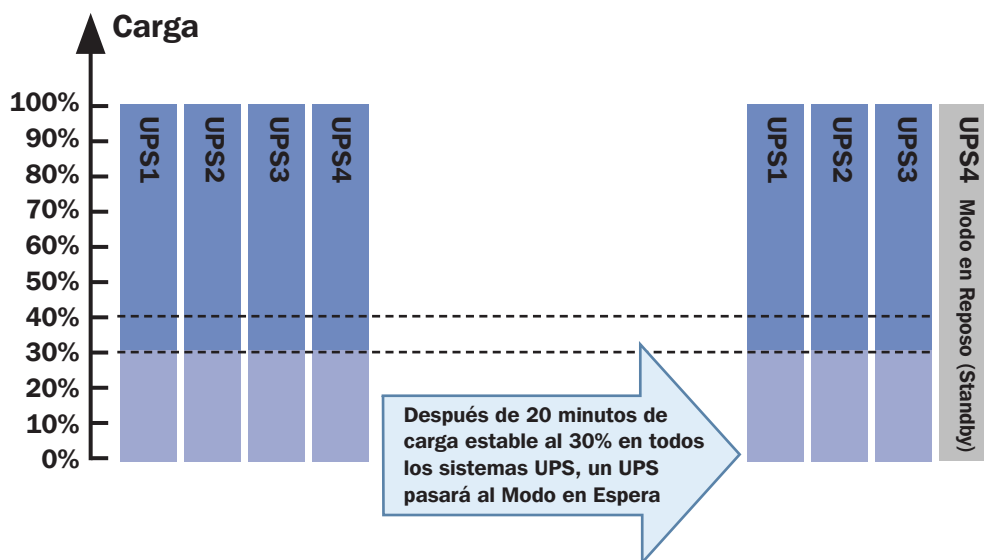
Figura 4-28D: Ejemplo, Modo en Reposo Inter con Cuatro Sistemas UPS
