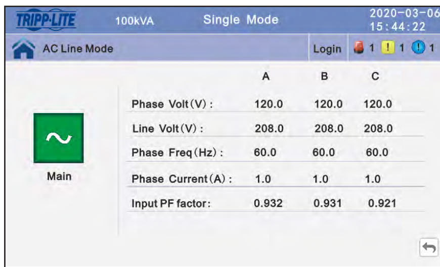
Figura 4-9: Ventana de Pantalla de Datos Principales
