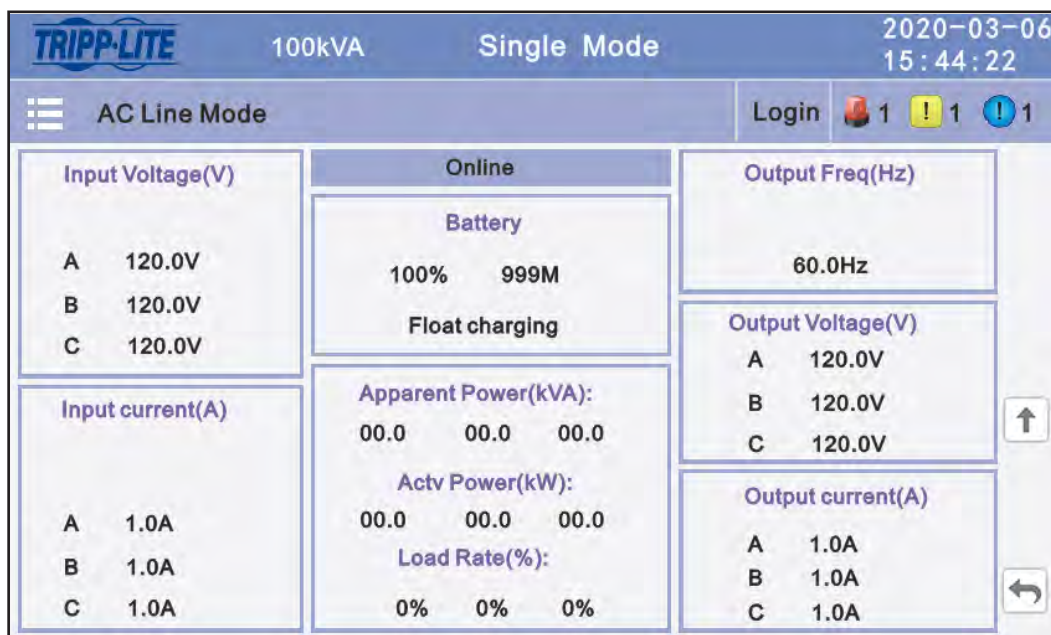
Figure 4-7B : Page principale 2 de l'écran ACL. (Appuyer sur l'icône Page arrière pour revenir à la page principale illustrée à la Figure 4-7A.)
