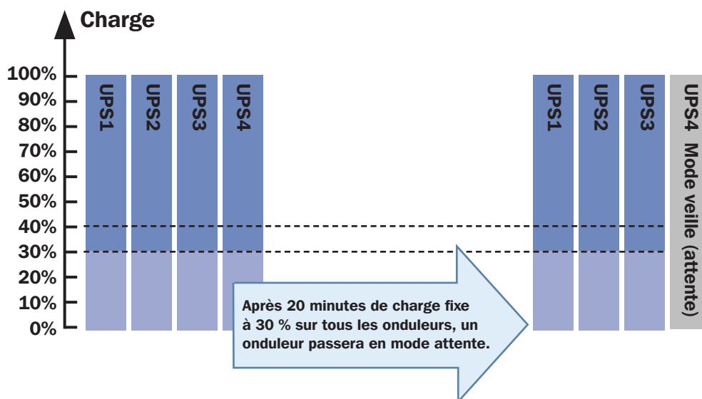
Figure 4-28D : Exemple de Inter Sleep Mode avec quatre onduleurs
