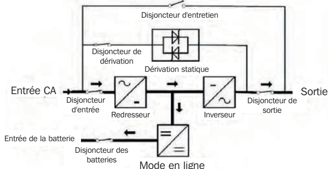
Figure 4-1 : Mode en ligne CA
