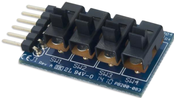
The PmodSWT.
