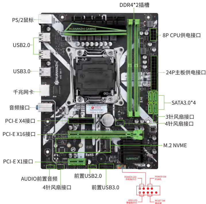
图1-1 X99-8M F主板图解
