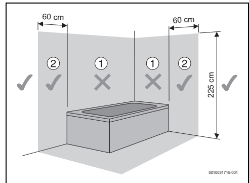
Fig. 8 Volume de protection
