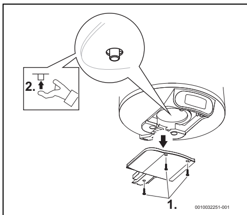
Fig. 12 Termostat de siguranță
