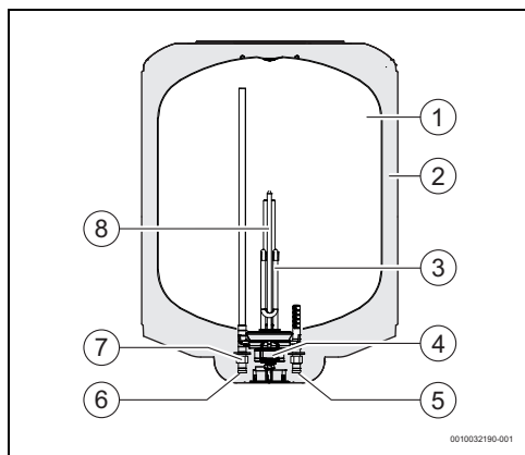
Sl.3 Komponente naprave
