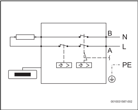
Мал. 13 Схема з'єднань
