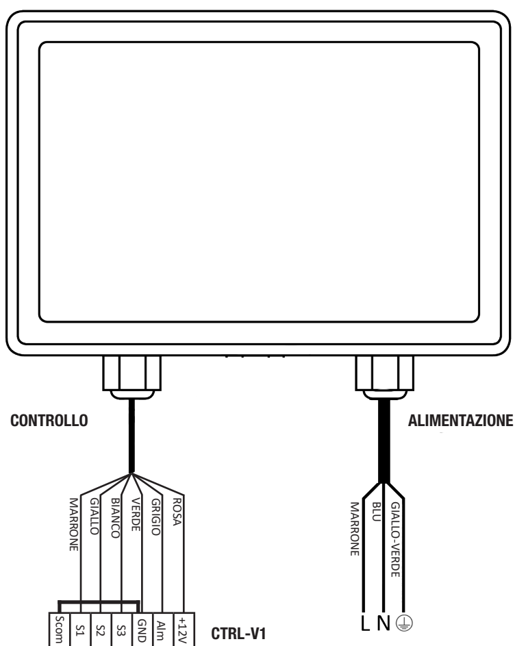
Fig. 5.h Precablaggio
