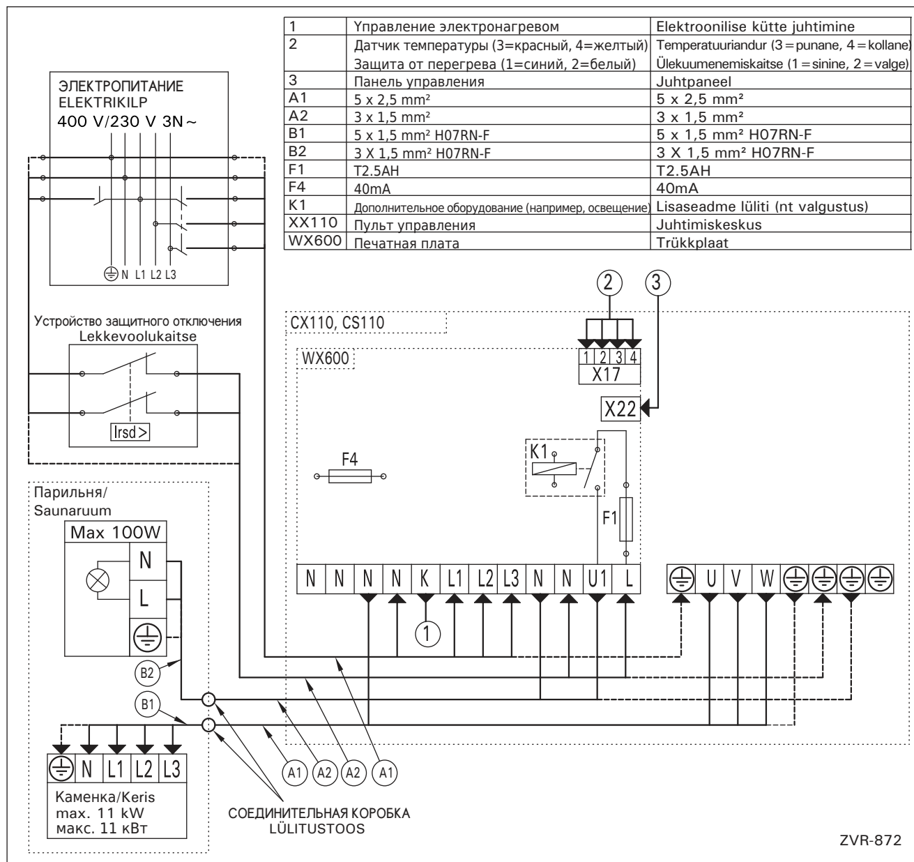
Рисунок 4. Электрические подключения Joonis 4. Elektriühendused
