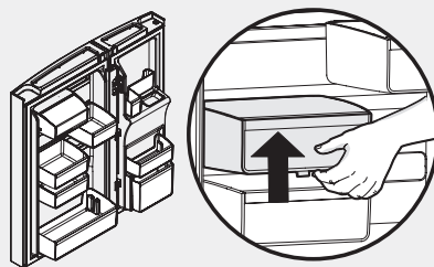
Custom Flex-Türbehälter
