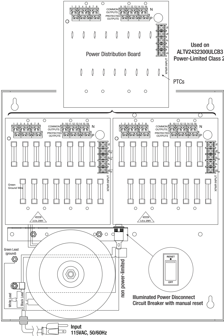
Fig. 1 - ALTV2432300UL3, ALTV2432300ULCB3
