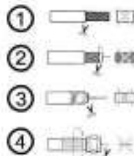
F Connector twist-on Connecteur F à visser Connettore F ad avvitamento
