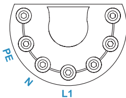
3 Ledninger: PE, Nøytral, Fase L1.
