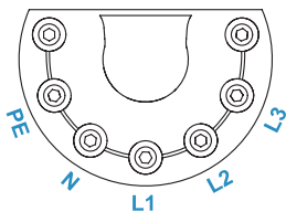
5 Ledninger: PE, Nøytral, Fase L1, L2, L3.
