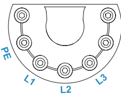
4 Ledninger: PE, Fase L1, L2, L3.
