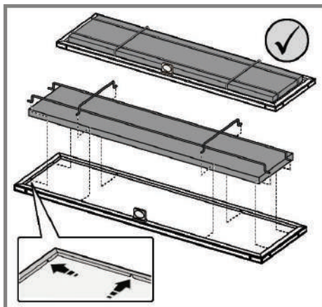
Filtre au charbon circulaire
