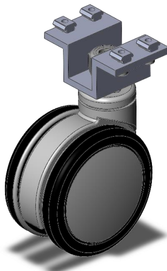
Fig. 5 Caster Module
