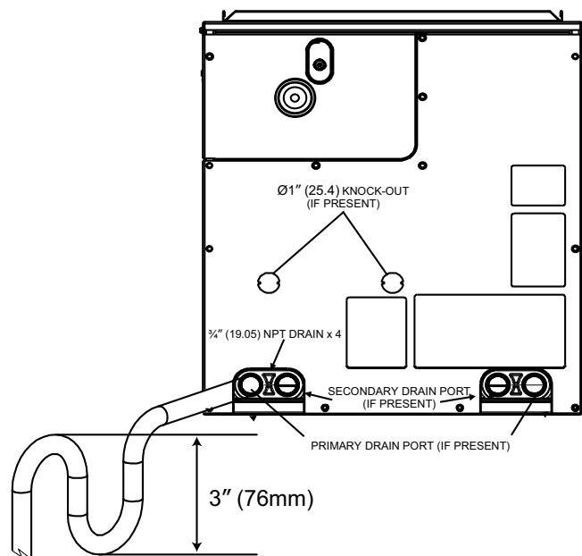
Fig. 8 – Condensate Trap
