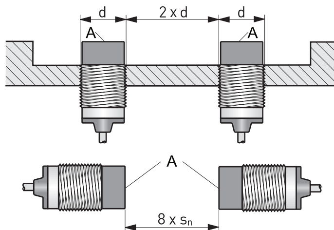
Figura 2: Resistenza meccanica
