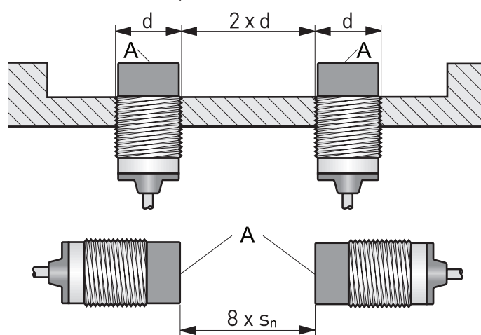
Figura 2: Robustez mecânica
