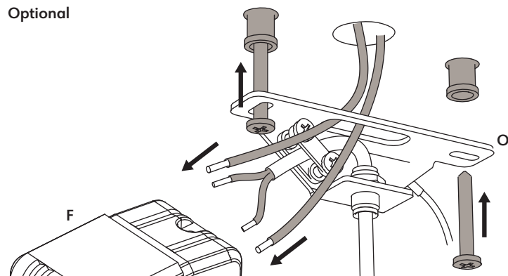
Wiring diagram Schema di collegamento
