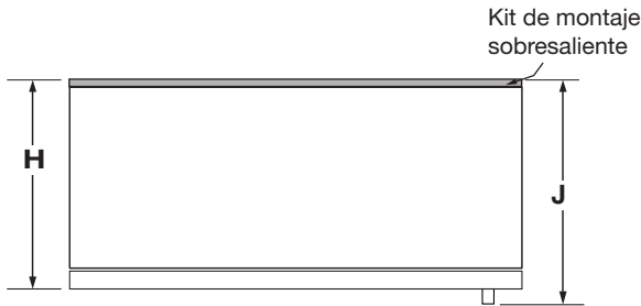
VISTA SUPERIOR CON KIT DE MONTAJE SOBRESALIENTE
