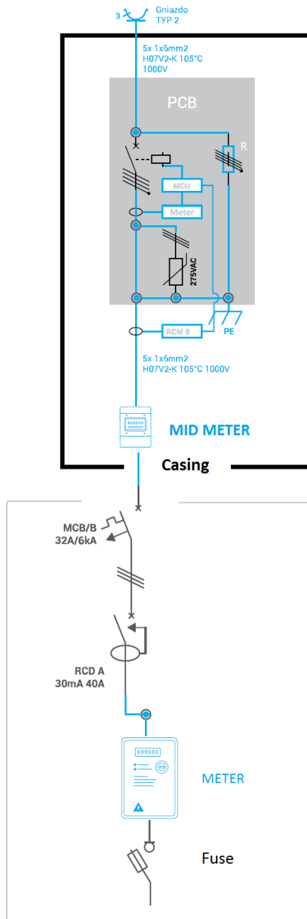
Fig. 14: Schematy wariantów podłączenia 2./2.
