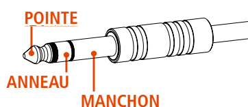
CONNECTEUR JACK (TRS) Câblage mono symétrique
