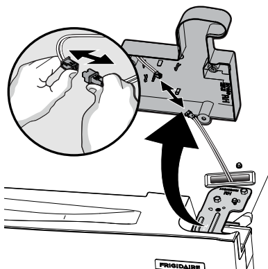
Right Door Dispenser Unit
