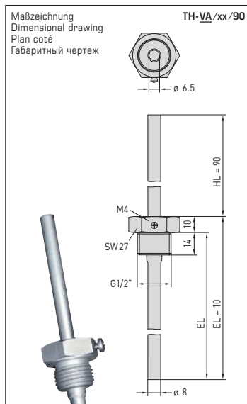
TH-VA/xx/90 Edelstahltauchhülse mit Halsrohr Stainless steel immersion sleeve with neck tube doigt de gant en acier inox avec tube prolongateur Гильза погружная из высококачественной стали с горловойной
