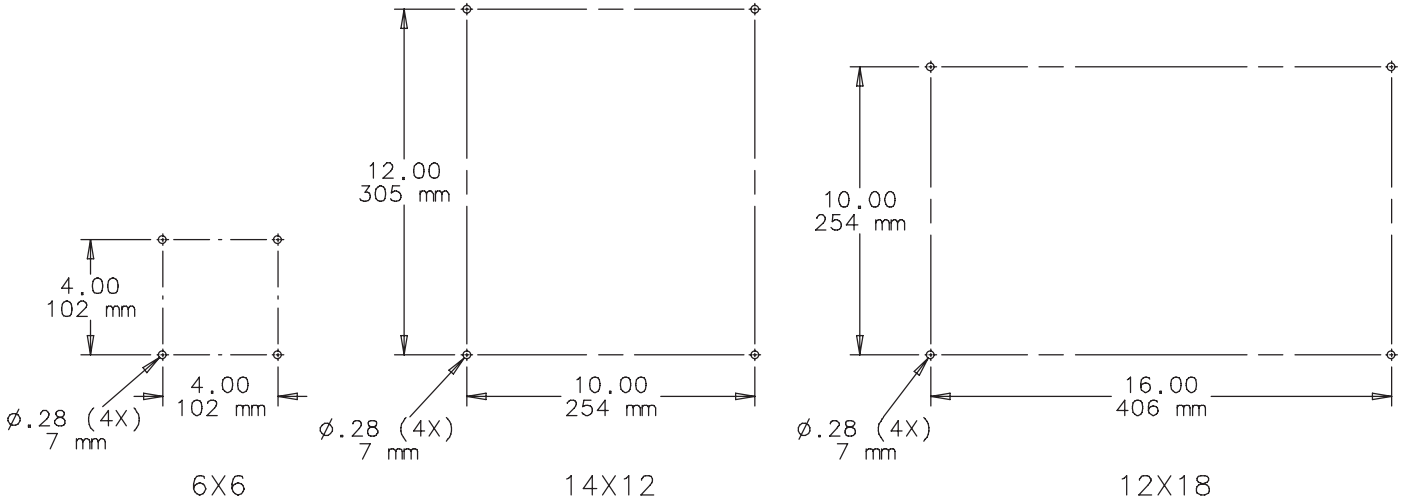
Mounting Pattern Modèle De Support Patrón Del Montaje
