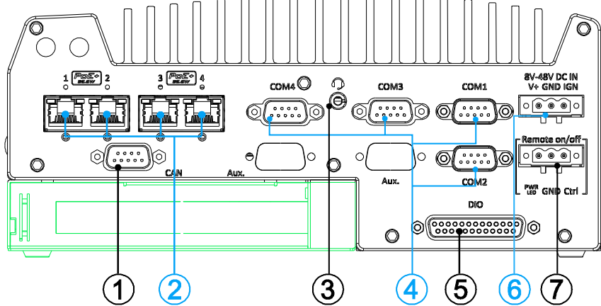
Nuvo-9204/ 9208VTC
